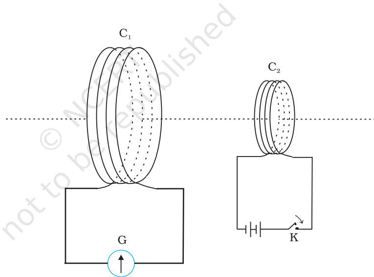
चित्र 6.3 प्रयोग 6.3 के लिए प्रयोगात्मक व्यवस्था
