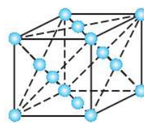
फलक-केंद्रित
