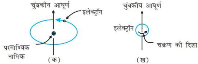
चित्र 1.35—(क) इलेक्ट्रॉन की कक्षीय गति,
