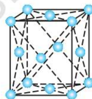
फलक-केंद्रित
