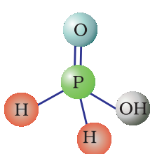
\text{H}_3\text{PO}_2 हाइपोफॉस्फोरस अम्ल
