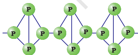
चित्र 7.3— लाल फ़ॉस्फोरस
