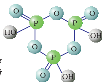
(\text{HPO}_3)_3 साइक्लोट्राइमेटाफॉस्फोरिक अम्ल
