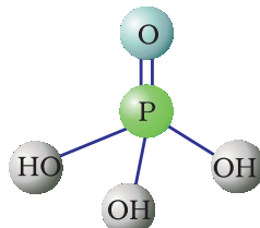
\text{H}_3\text{PO}_4 आर्थोफॉस्फोरिक अम्ल
