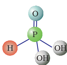
\text{H}_3\text{PO}_3 आर्थोफॉस्फोरस अम्ल
