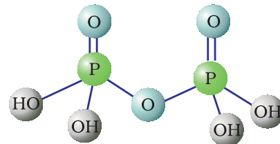
\text{H}_4\text{P}_2\text{O}_7 पायरोफॉस्फोरिक अम्ल
