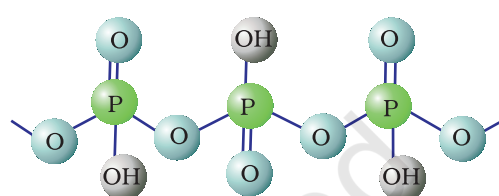
(\text{HPO}_3)_3 पॉलीमेटाफॉस्फोरिक अम्ल
