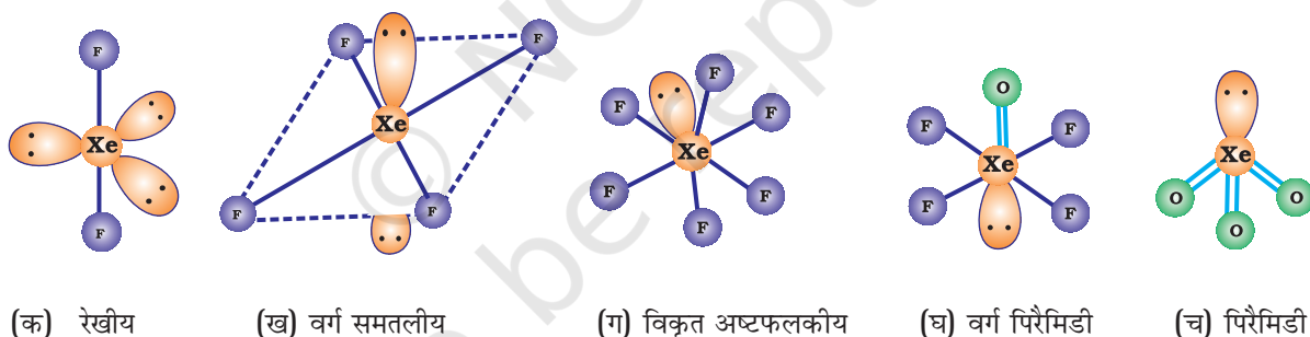
चित्र 7.9— (क) \text{XeF}_2 , (ख) \text{XeF}_4 , (ग) \text{XeF}_6 , (घ) \text{XeOF}_4 तथा (च) \text{XeO}_3 की संरचनाएं
