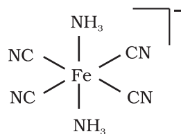
विपक्ष समावयव
