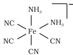
समपक्ष समावयव
