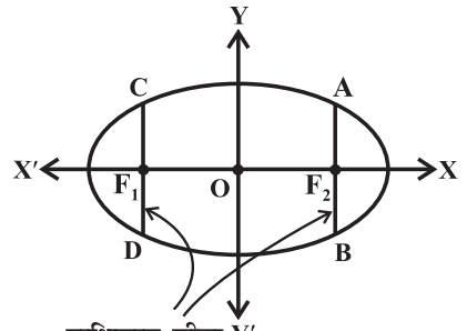
नाभिलंब जीवा Y' आकृति 11.28
