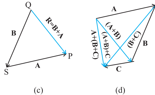
चित्र 4.3 (a) सदिश \mathbf{A} तथा 2\mathbf{A} , (b) सदिश \mathbf{A} व -\mathbf{A} का ग्राफी विधि द्वारा जोड़ना, (c) सदिशों \mathbf{B} व \mathbf{A} का ग्राफी विधि द्वारा जोड़ना, (d) सदिशों के जोड़ से संबंधित साहचर्य नियम का प्रदर्शन।
