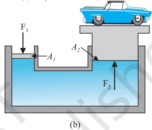
चित्र 10.6 (b) द्रव चालित उत्थापक, भारी बोझ उठाने की एक युक्ति के कार्य करने के सिद्धांत की व्याख्या का योजनाबद्ध आरेख।
