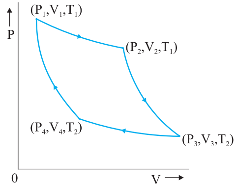
चित्र 12.11 किसी ऊष्मा इंजन के लिए कानों चक्र जिसमें कार्यकारी पदार्थ के रूप में आदर्श गैस का उपयोग होता है।
