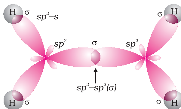
चित्र 13.4 एथीन का कक्षीय आरेख केवल \sigma बन्धों को चित्रित करते हुए
