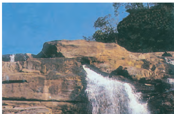
चित्र 2-6 : प्रायद्वीपीय पठार
