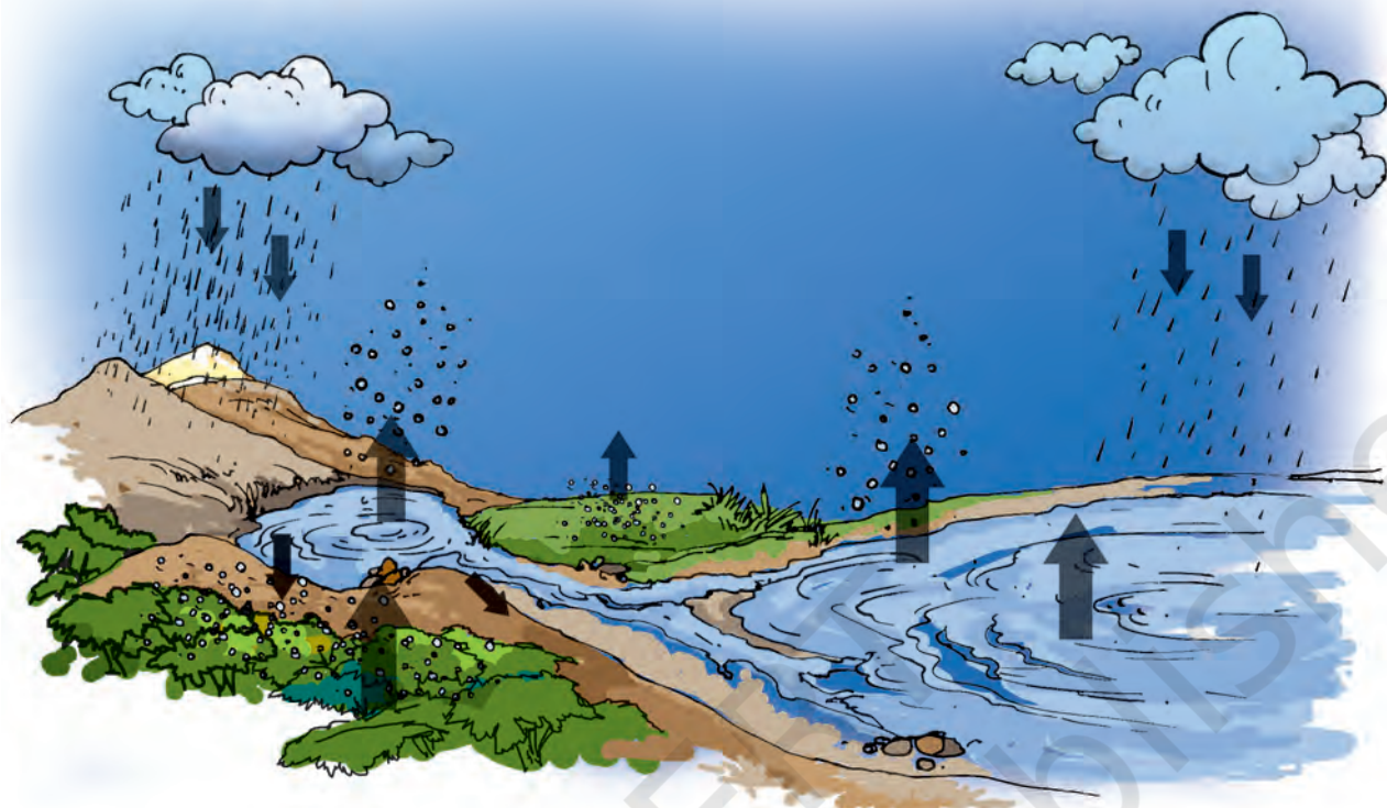
चित्र 14.9 जलचक्र
