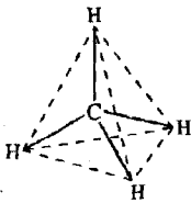
चतुष्फलकीय ज्यामिति
