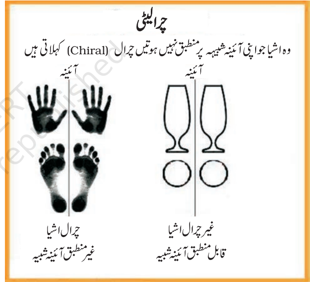
شکل 10.4: چرال (Chiral) اور غیر چرال (Achiral) اشیا کی کچھ عام مثالیں
