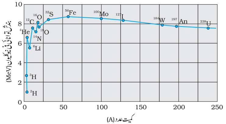
شکل 13.1: بندش توانائی فی نیوکلون بہ طور تفاعل کمیت عدد
