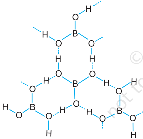
شکل 11.1 بورک ایسڈ کی ساخت : نقطہ دار خطوط ہائڈروجن بند کو ظاہر کرتے ہیں۔
