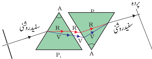
شکل 11.6 سفید روشنی کے اسپیکٹرم کا باز تراحد
