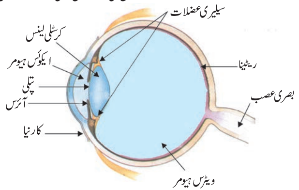
شکل 11.1 انسانی آنکھ
