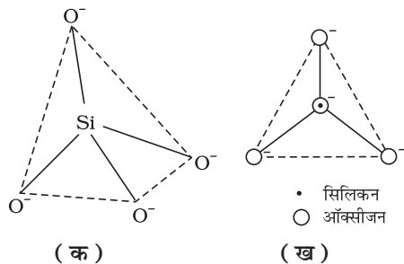
चित्र 11.7 : (क) \text{SiO}_4^{4-} ऋणायन की चतुष्फलक संरचना (ख) \text{SiO}_4^{4-} इकाई का निरूपण
