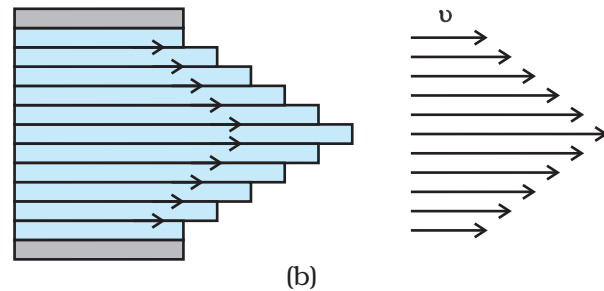
चित्र 10.14 (a) दो समांतर काँच की प्लेटों के बीच रखे द्रव की एक परत जिसमें काँच की निचली प्लेट स्थिर है तथा ऊपरी प्लेट \nabla वेग से दाहिनी ओर गतिमान है। (b) पाइप में श्यान प्रवाह के लिए वेग वितरण।
