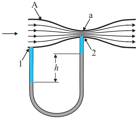
चित्र 10.11 वेंदुरीमापी का व्यवस्था आरेख।
