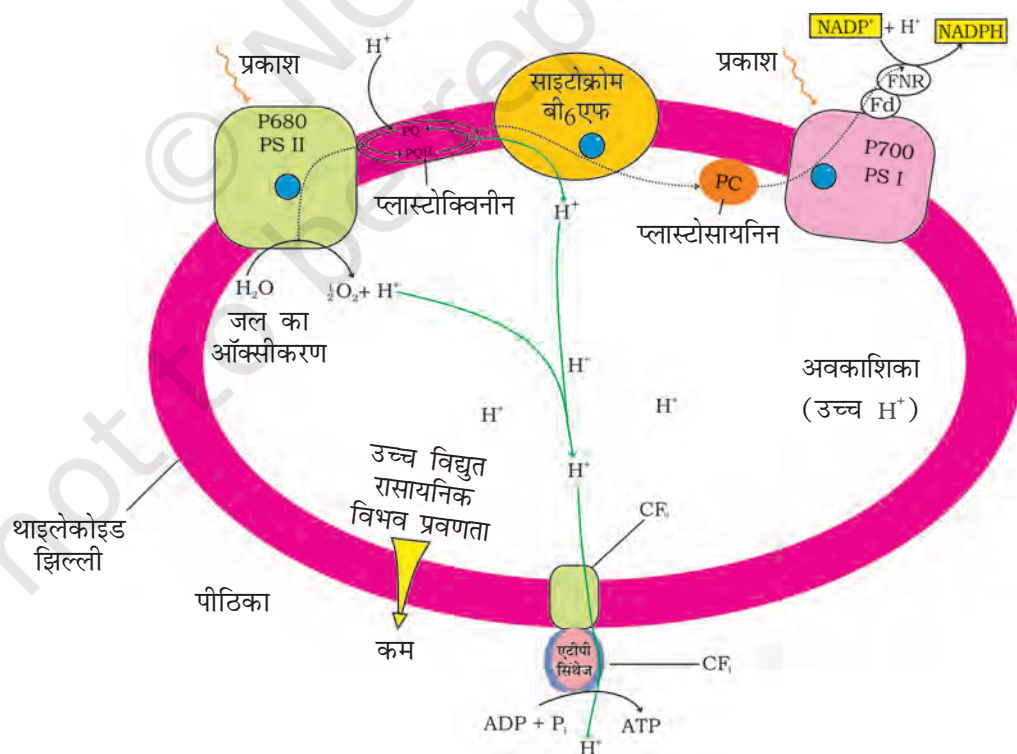
चित्र 13.7 रसोपरासरण के द्वारा एटीपी का निर्माण
