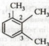
1, 2, 3-Trimethylbenzene
