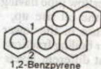
1,2-Benzpyrene
