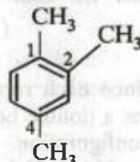
1, 2, 4-Trimethylbenzene
