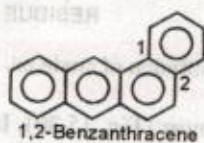
1,2-Benzanthracene
