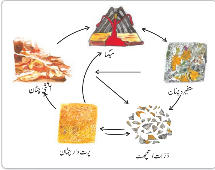
شکل 2.4 چٹانی گردش
