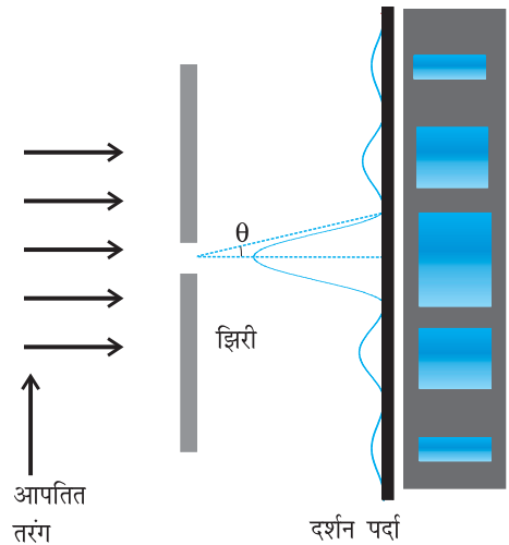
चित्र 10.16 एकल झिरी द्वारा विवर्तन के लिए फ्रिंजों का फ़ोटोग्राफ़ तथा तीव्रता वितरण।
