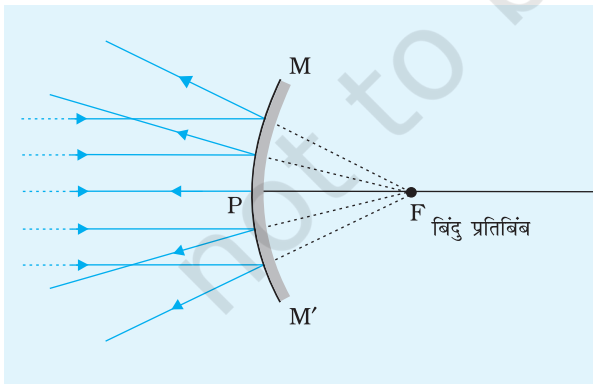
चित्र E 11.1(a) बिंब अनंत पर स्थित है। उत्तल दर्पण के पीछे एक अत्यधिक छोटा बिंदु प्रतिबिंब प्राप्त होता है।
