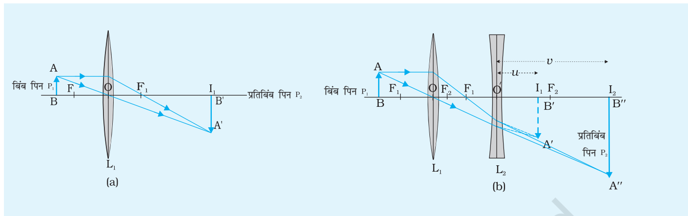
चित्र E 12.2 (a) उत्तल लेंस तथा (b) उत्तल लेंस तथा अवतल लेंस के संयोजन द्वारा प्रतिबिंब बनना
