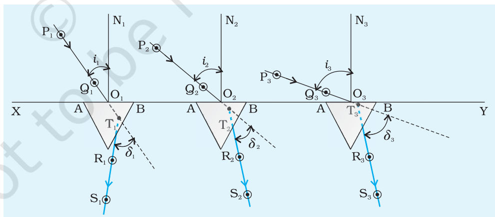
चित्र E 13.2 विभिन्न आपतन कोणों के लिए काँच के प्रिज्म से प्रकाश का अपवर्तन
