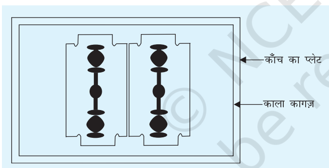
चित्र A12.1 दो रेज़र ब्लेडों एक काँच का स्लाइड तथा काले कागज़ के उपयोग से बनी एक संकीर्ण झिरी
