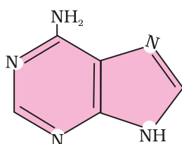
एडेनिन (प्यूरीन)
