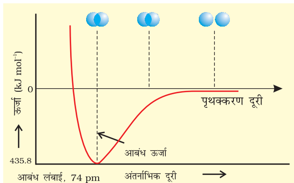
चित्र 4.8: H_2 अणु के विरचन के लिए H परमाणुओं के बीच अंतराणु दूरी की सापेक्ष स्थितिज ऊर्जा का आरेख, आरेख में न्यूनतम ऊर्जा स्थिति H_2 की सर्वाधिक स्थायी अवस्था दर्शाती है।
