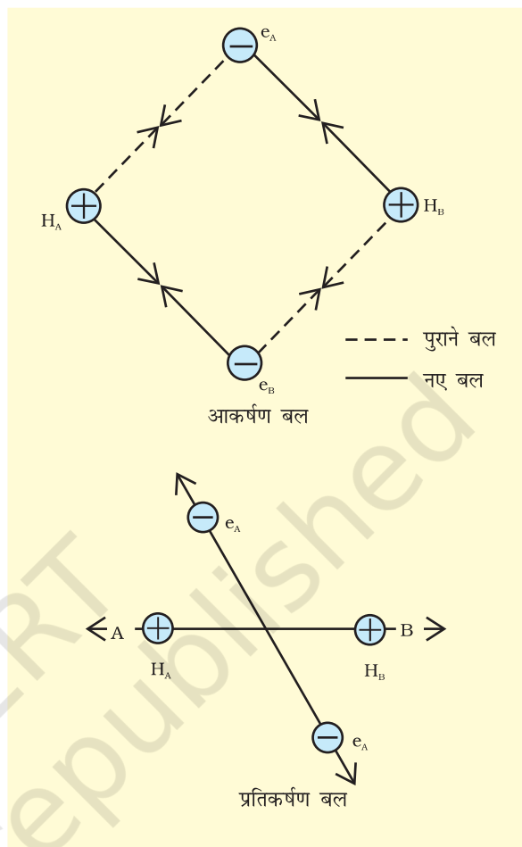
चित्र 4.7 H_2 अणु के विचरण में आकर्षण तथा प्रतिकर्षण बल
