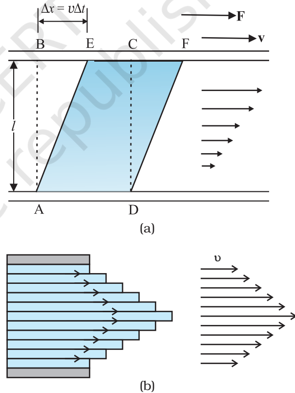
चित्र 10.14 (a) दो समांतर काँच की प्लेटों के बीच रखे द्रव की एक परत जिसमें काँच की निचली प्लेट स्थिर है तथा ऊपरी प्लेट \nabla वेग से दाहिनी ओर गतिमान है। (b) पाइप में श्यान प्रवाह के लिए वेग वितरण।
