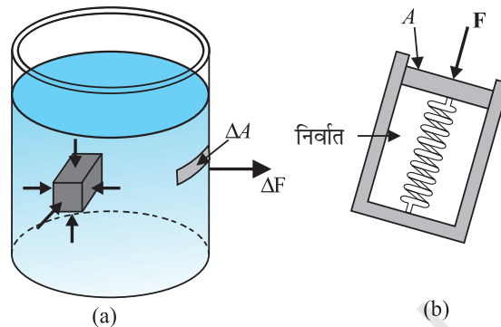
चित्र 10.1 (a) बीकर के द्रव में डूबे पिण्ड अथवा उसकी दीवारों पर द्रव द्वारा आरोपित बल पिण्ड के पृष्ठ के हर बिंदु के लंबवत् कार्य करता है। (b) दाब मापने के लिए युक्ति का आदर्श रूप।
