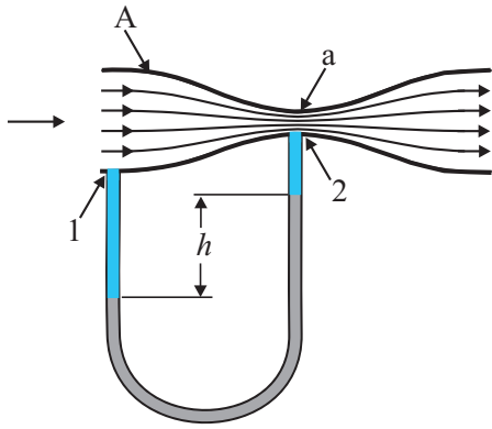
चित्र 10.11 वेंचुरीमापी का व्यवस्था आरेख।
