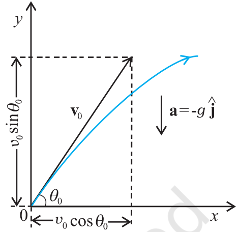
شکل 4.17 ایسی شے کی حرکت جسے زاویہ \theta_0 پر، رفتار \vec{v}_0 کے ساتھ پھینکا (اچھالا) گیا ہے۔
