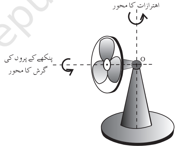
شکل (b) 7.5 اہتراز کرتا ہوا میٹر کا پنکھا مع گردش پر۔ پنکھے کی دھوری نقطہ O جامد ہے۔ پنکھے کے پر گردش حرکت کر رہے ہیں۔ جبکہ پنکھے کے پروں کا گردش محور اہترازی حرکت کر رہا ہے۔
