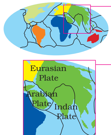
Fig. 15.10 : Earth plates
