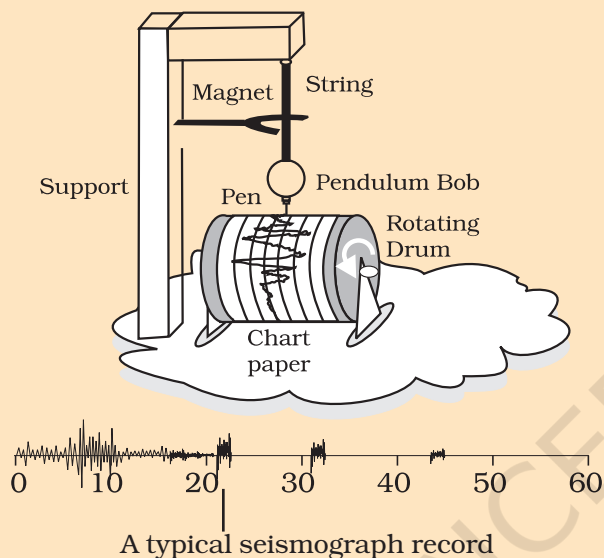
Fig. 15.13 : A seismograph
