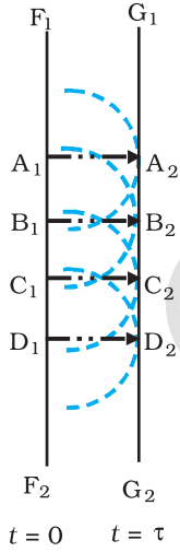
चित्र 10.3 दाईं ओर संचरित होने वाली एक समतल तरंग के लिए हाइगेंस का ज्यामितीय निर्माण। F_1F_2 , t = 0 पर एक समतल तरंगाग्र है तथा G_1G_2 t समय बाद का एक तरंगाग्र है। रेखाएँ A_1A_2 , B_1B_2 ... आदि F_1F_2 तथा G_1G_2 दोनों के लंबवत हैं तथा किरणों को निरूपित करती हैं।
