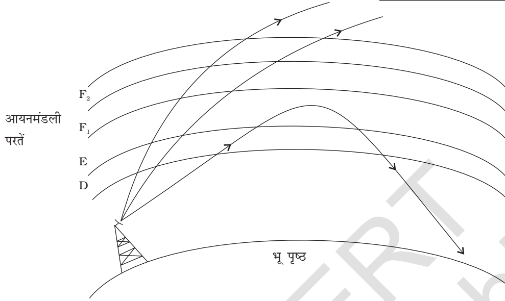
चित्र 15.4 व्योम तरंग संचरण। सारणी 15.3 में परतों का नामकरण दिया गया है।
