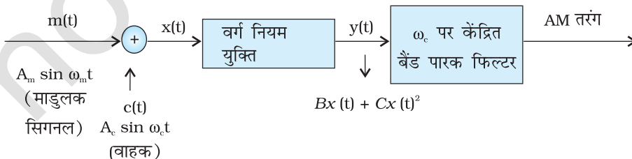
चित्र 15.10 AM सिग्नल प्राप्त करने के लिए सरल माडुलक का ब्लॉक आरेख।
