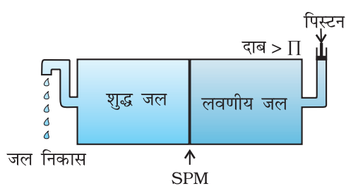
चित्र 2.11— जब विलयन पर परासरण दाब से अधिक दाब लगाया जाता है तो प्रतिलोम परासरण होता है।
