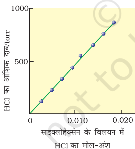
चित्र 2.2— \text{HCl} गैस की साइक्लोहेक्सेन में 293\text{ K} पर विलेयता के प्रायोगिक परिणाम। रेखा का ढाल हेनरी स्थिरांक K_H को व्यक्त करता है।
