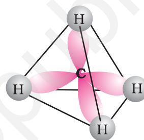
चित्र 13.1 मेटेन ( \text{CH}_4 ) की चतुष्फलक संरचना
