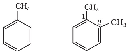
मेथिल बेन्जीन (टॉलूईन)
