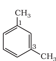
1, 3-डाइमेथिलबेन्जीन (m-जाइलीन)
