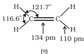
चित्र 13.5 एथीन का कक्षीय आरेख (क) \pi आबंध बनना (ख) \pi -अभ्र का बनना तथा (ग) आबंध कोण तथा आबंध लंबाई
