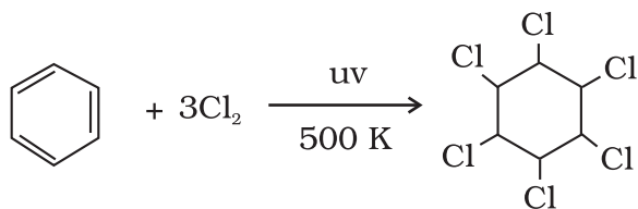
बेन्जीनहेक्साक्लोराइड (13.81)
