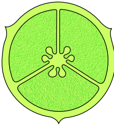
स्तंभीय बीजांडन्यास
