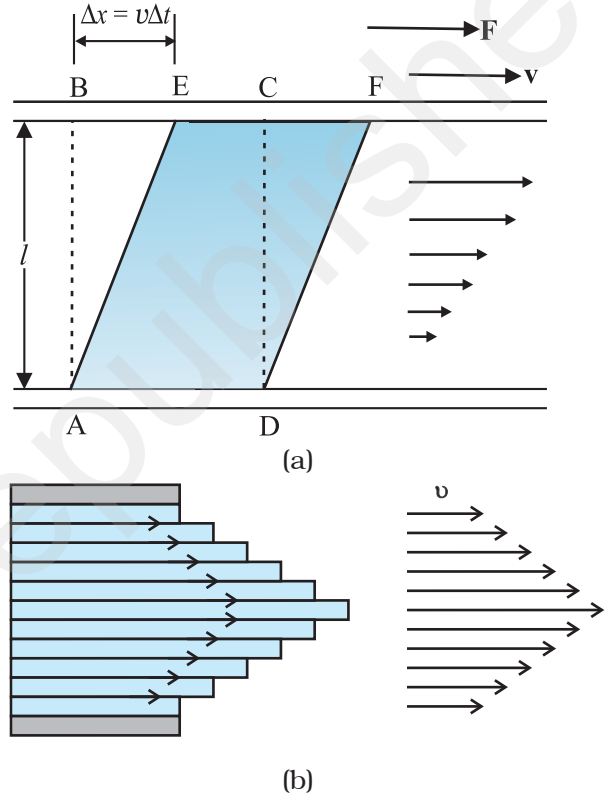
चित्र 10.14 (a) दो समांतर काँच की प्लेटों के बीच रखे द्रव की एक परत जिसमें काँच की निचली प्लेट स्थिर है तथा ऊपरी प्लेट \mathbf{v} वेग से दाहिनी ओर गतिमान है। (b) पाइप में श्यान प्रवाह के लिए वेग वितरण।
