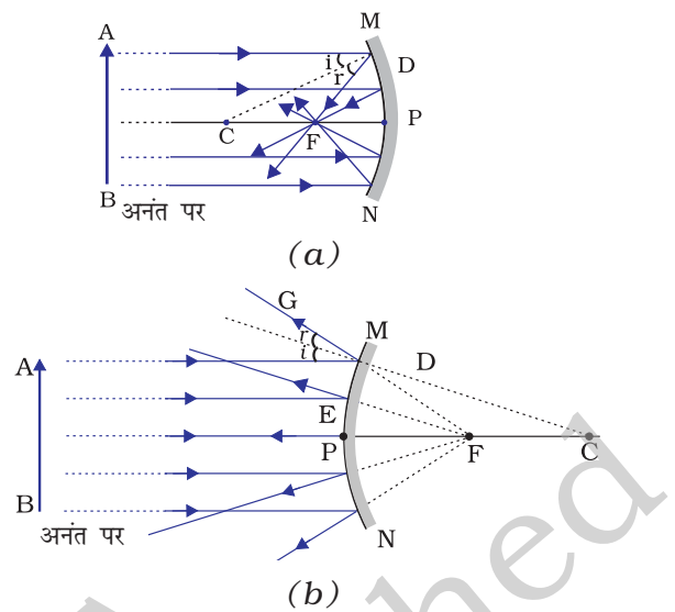
चित्र 10.2 (a) अवतल दर्पण (b) उत्तल दर्पण
