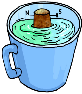
شکل 13.12 کپ میں کمپاس
