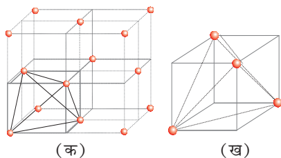
चित्र 1- (क) ccp संरचना के प्रति एकक कोष्ठिका में 8 चतुष्फलकीय रिक्तियाँ (ख) एक चतुष्फलकीय रिक्ति ज्यामिती प्रदर्शित करते हुए।
