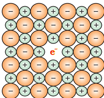
चित्र 1.32 – क्रिस्टल में एक F- केंद्र
