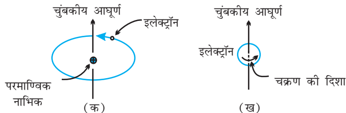
चित्र 1.35—(क) इलेक्ट्रॉन की कक्षीय गति,
