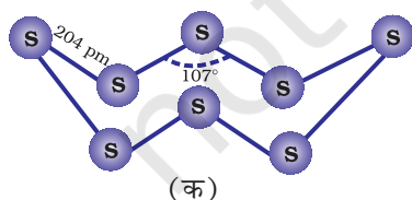
चित्र 7.5 (क) विषमलंबाक्ष सल्फर में S_8 वलय
