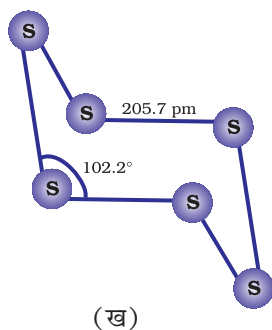
चित्र 7.5 (ख) साइक्लो S_6 रूप संरचनाएँ
