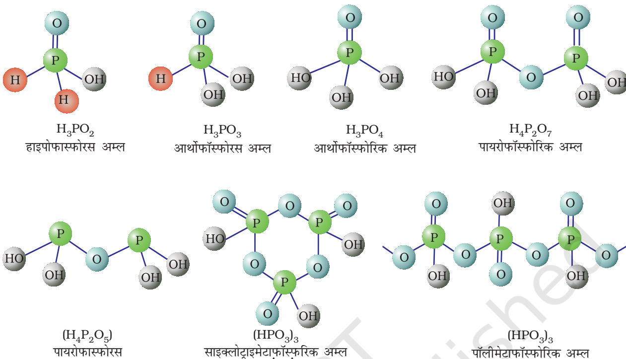
चित्र 7.4—फॉस्फोरस के कुछ प्रमुख आक्सोअम्लों की संरचनाएँ
