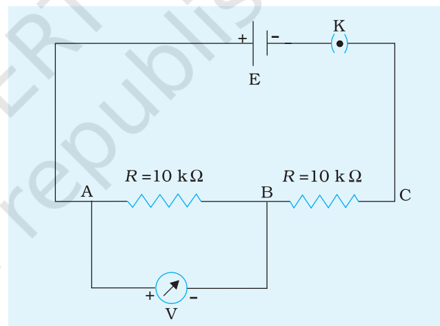
चित्र D 7.1 वोल्टमीटर का प्रतिरोध मापना
