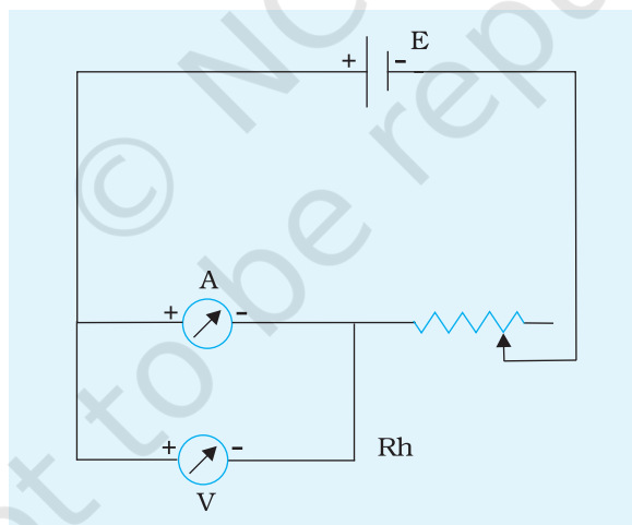
चित्र D 6.1 ऐमीटर के प्रतिरोध की माप
