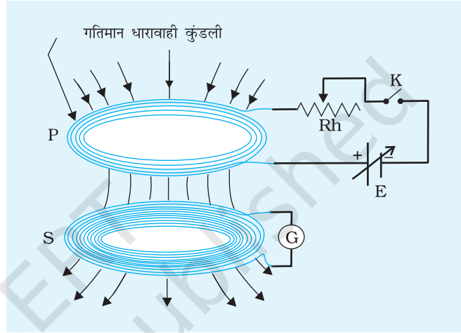
चित्र D 12.2 गतिमान धारावाही कुंडली P कुंडली S में प्रेरित emf उत्पन्न करती है।
