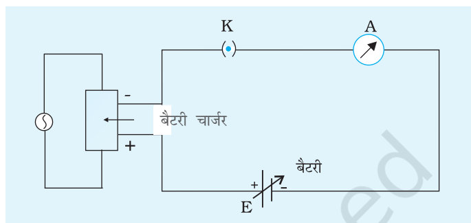
चित्र D 5.2 बैटरी चार्जक की सहायता से बैटरी के चार्जिंग के लिए परिपथ
