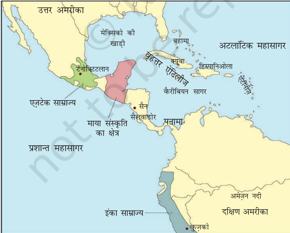
मानचित्र 1: मध्य अमरीका और कैरीबियन द्वीपसमूह।
