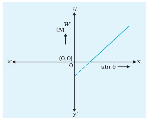
चित्र E 8.3 W तथा \sin \theta के बीच ग्राफ
