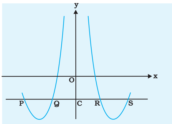
चित्र P 2.2 गुरुत्व केंद्र से दूरी तथा दोलन काल के बीच ग्राफ
