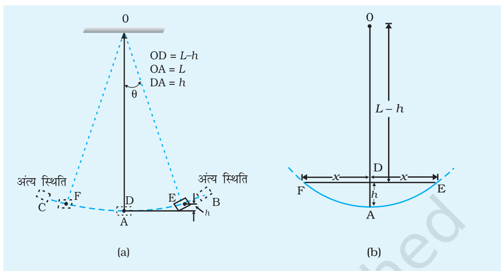
चित्र P1.1 एक दोलाचमान लोलक
