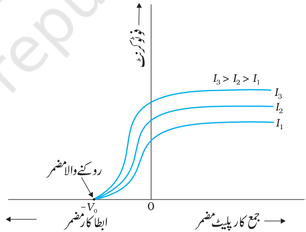
شکل 11.3: واقع اشعاع کی مختلف شدتوں کے لیے جمع کار پلیٹ مضمّر کے ساتھ فوٹو کرنٹ کی تبدیلی
