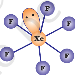
(c) مسخ شدہ آکٹا ہیڈرل
