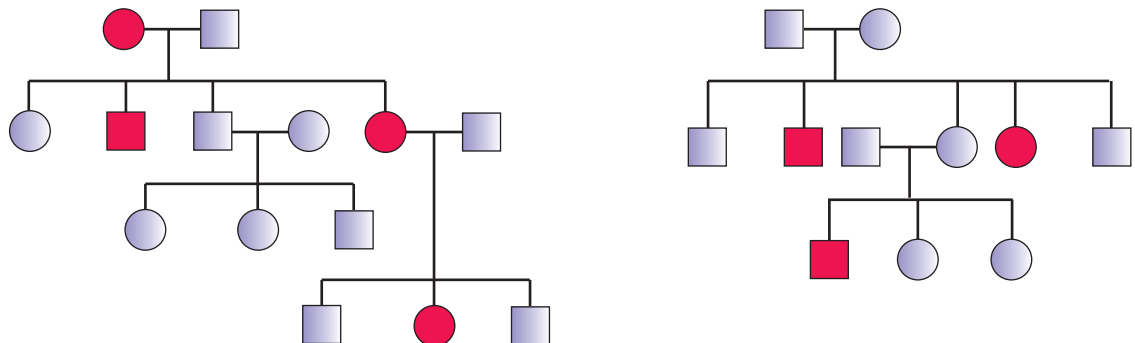
شکل 5.14 (a) آٹوسومل ڈامینیٹ صفت (مثلاً مائوٹانک ڈسٹرونی) (b) آٹوسومل ریسو صفت (مثلاً سیل انیمیا) کی پیڈیگری تجزیے کا نمونہ۔
