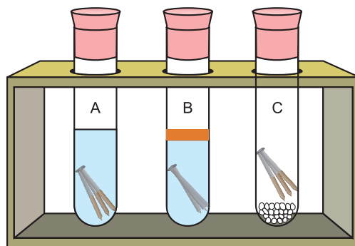
चित्र 3.1 : (a) जल में डूबी लोहे की कीलें; (b) उबले हुए आसुत जल में डूबी लोहे की कीलें जिसमें से विलीन वायु निष्कासित कर दी गई हो तथा (c) शुष्क वायु में रखी लोहे की कीलें
