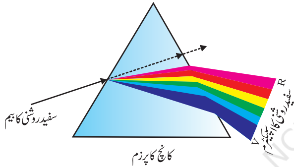
شکل 11.5 گلاس کے پرمز کے ذریعہ سفید روشنی کا انکسار
