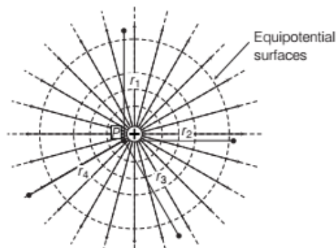
Equipotential surfaces for a point charge
